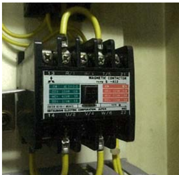
マグネットスイッチ
